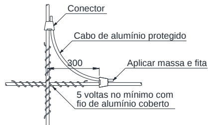
Figura 87 – Amarrações e ligações – Cruzamento aéreo
