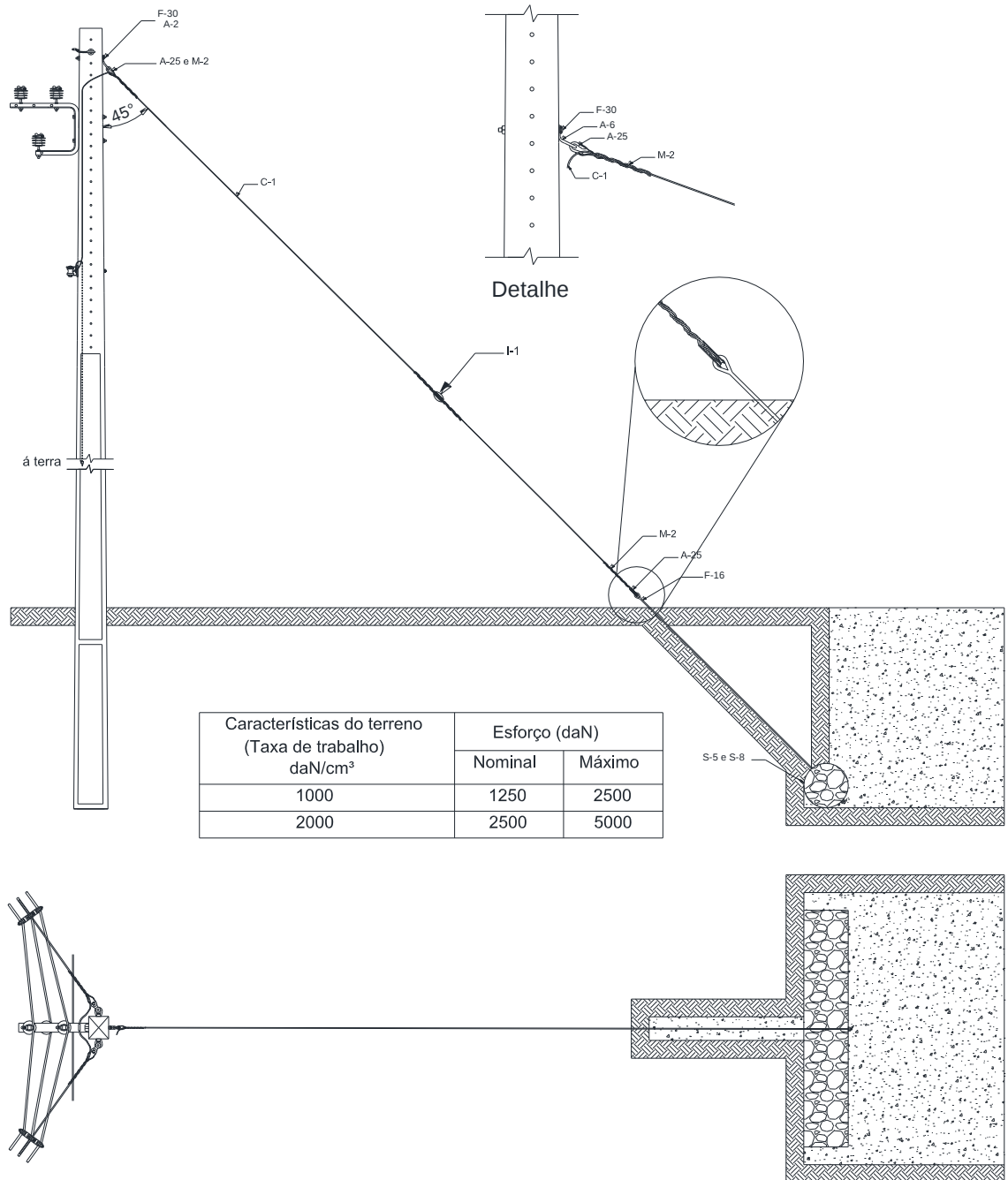
Figura 68 – Estaíamento – Estai de âncora
