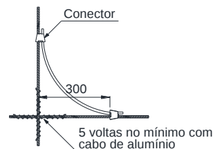
Detalhe da conexão do cabo mensageiro
