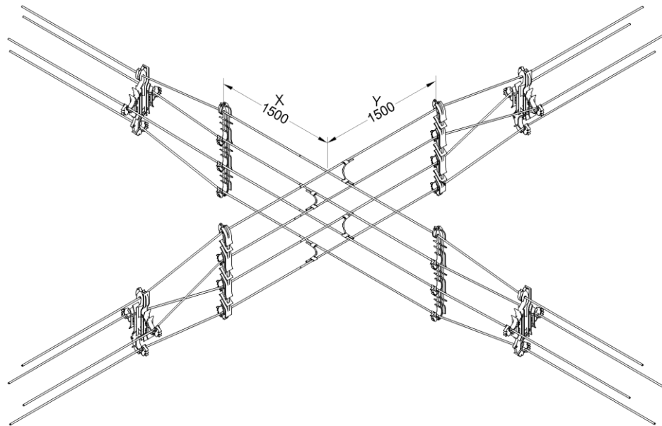
Detalhe da conexão dos cabos protegidos
