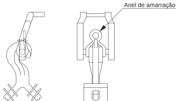
Figura 83 – Amarrações e ligações – Amarração do espaçador monofásico, vertical e losangular em estribo –
