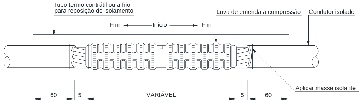
Figura 95 – Conexões e emendas – Emenda de cabo de alumínio protegido – Construção
